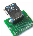
Módulo Adaptador USB Fêmea 3.0 para DIP
