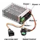
Controlador de Velocidade 10-50V 40A 2000W PWM com Chave Reversão
